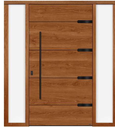
Modelo 240 Madera: Roble Color: Tinte Roble Tirador: CH-110 Perfil: Kitan® Negro + Abatible. Dos fijas laterales.
